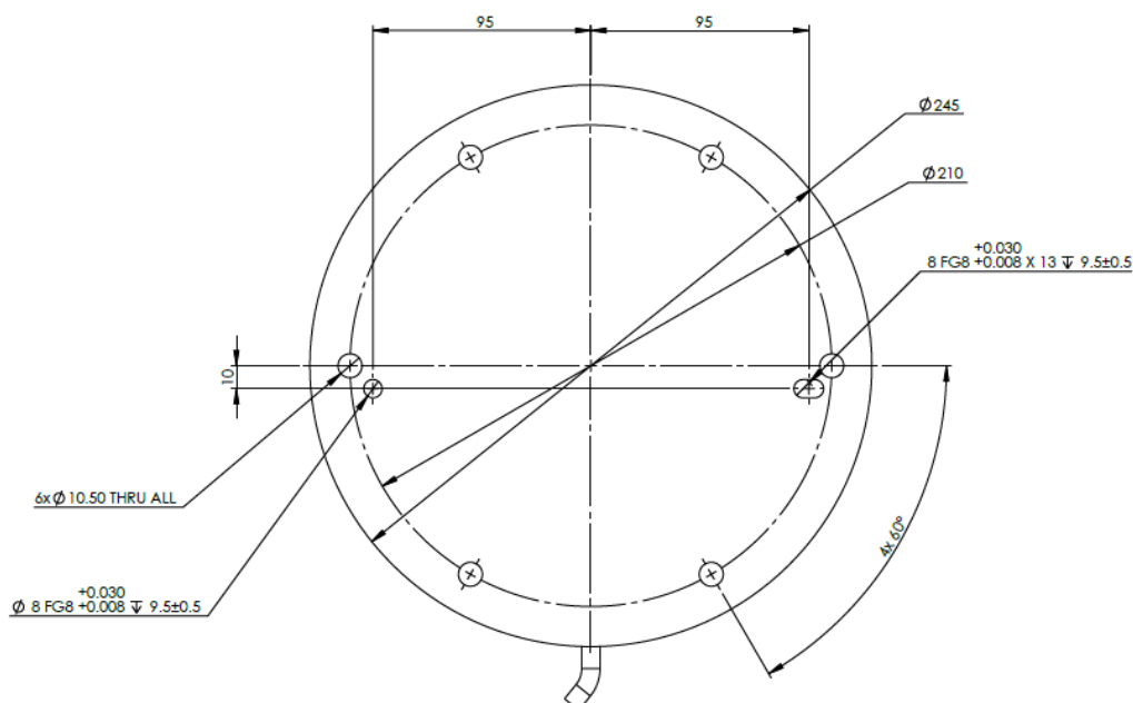
1.1: A robot alapjának alulnézete
